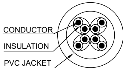
A-A 10:1
